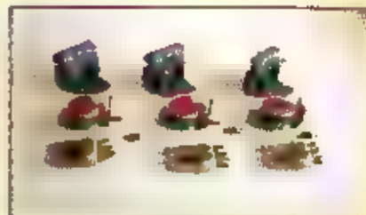
Foto 2. De in stap 1 gesloopte relais-onderdelen.
